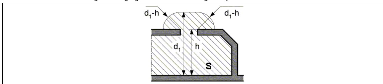
Figuur 2.5. Genaakbaarheidsgabarit: materiële elementen die het verplaatsingsoppervlak begrenzen hebben openingen die geen doorgang verlenen aan een lange staaf van 12 mm diameter
