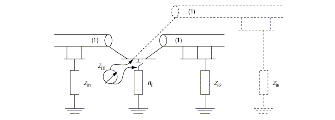
Figuur 2.10. Lusimpedantie van een aardverbinding Z_{EB}
