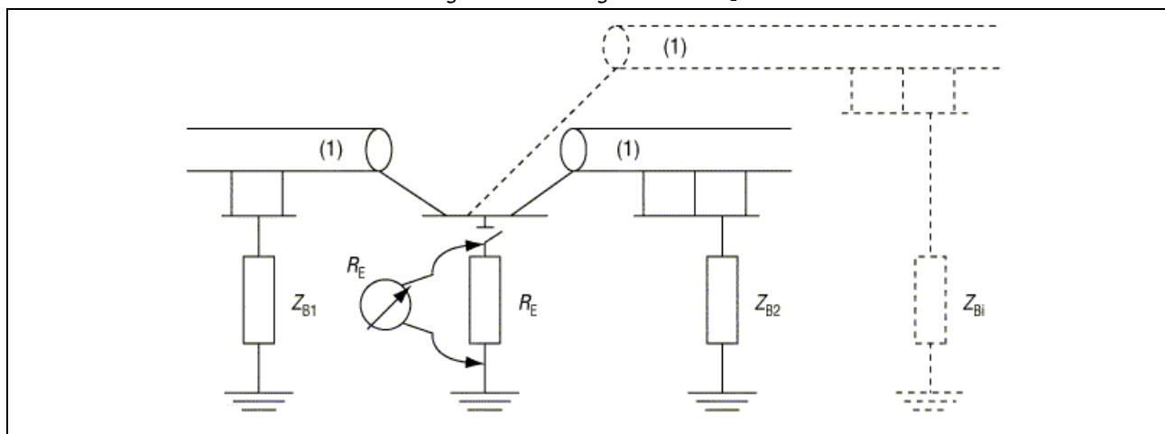
Figuur 2.7. Aardingsweerstand R_E
