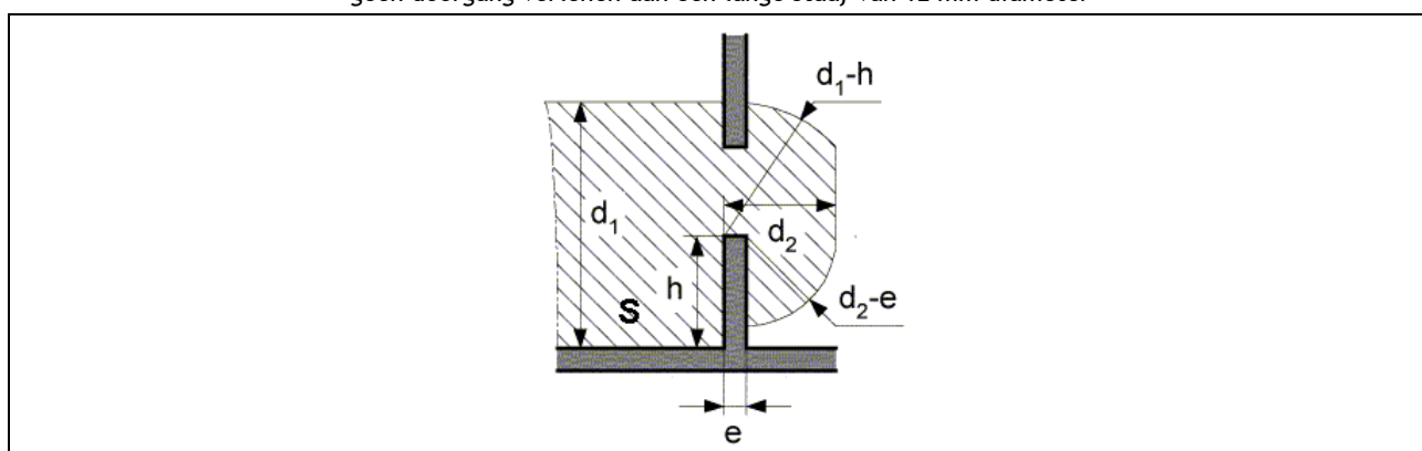
Figuur 2.4. Genaakbaarheidsgabarit: materiële elementen die het verplaatsingsoppervlak begrenzen hebben openingen die geen doorgang verlenen aan een lange staaf van 12 mm diameter
