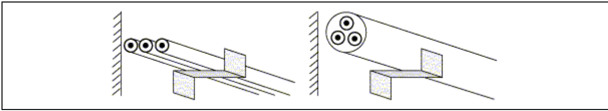
Figuur 5.6. Plaatsingswijzen van elektrische leidingen – Haken
