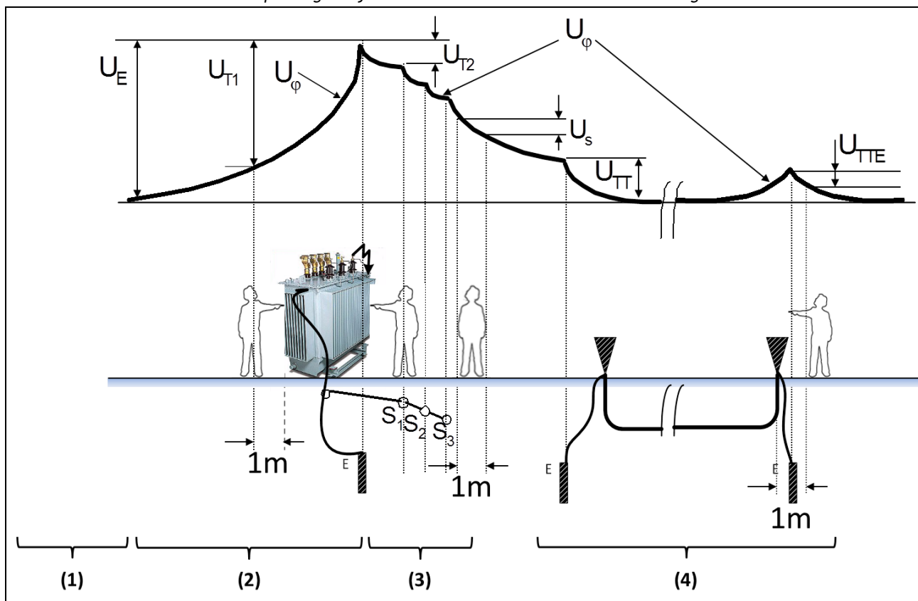
Figuur 2.6. Voorbeeld van verandering van aardbodemspanning en van spanningen bij het vloeien van stroom in de aardverbindingen
