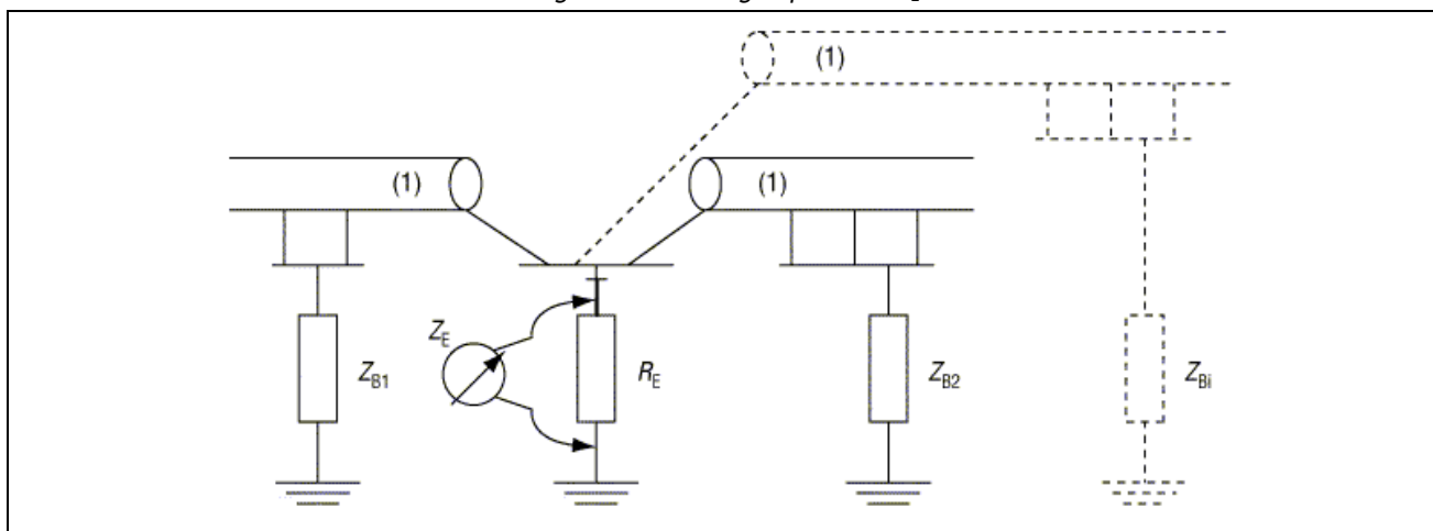
Figuur 2.8. Aardingsimpedantie Z_E
