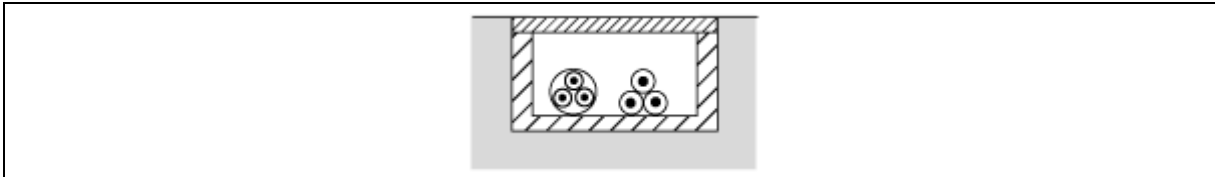
Figuur 5.8. Plaatsingswijzen van elektrische leidingen – Rechtstreekse plaatsing in gesloten kabelkanalen
