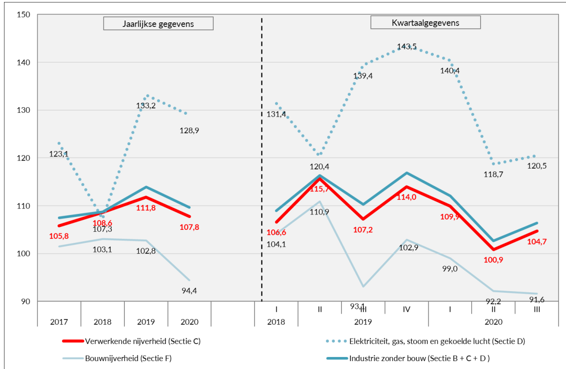
Grafiek 7. Evolutie van de industriële productie-indexen 2015 = 100.
