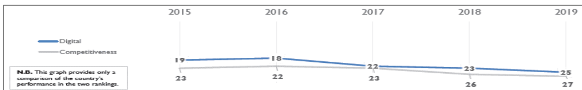
Grafiek 1. Concurrentievermogen en digitale rangschikking
