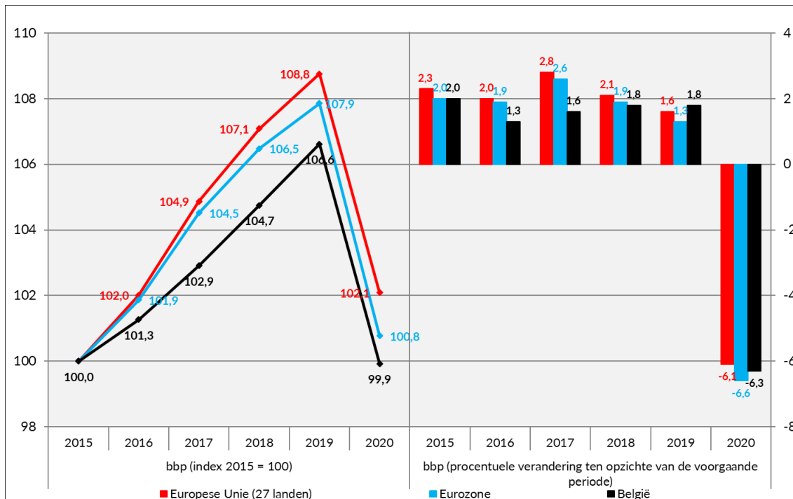
Grafiek 17. Bbp in België, in de Europese Unie en in de eurozone
