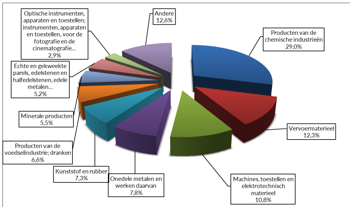
Grafiek 14. Uitsplitsing per sector van de Belgische goederenimport in 2020
