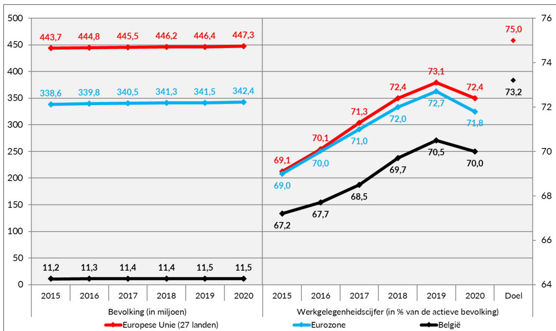
Grafiek 19. Bevolking en tewerkstelling
