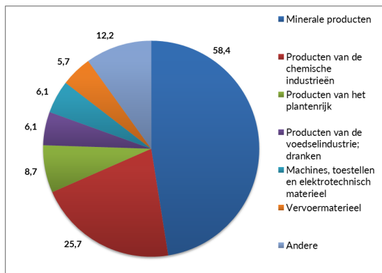
Grafiek 15. Uitvoer naar Angola in 2020 In miljoen euro.
