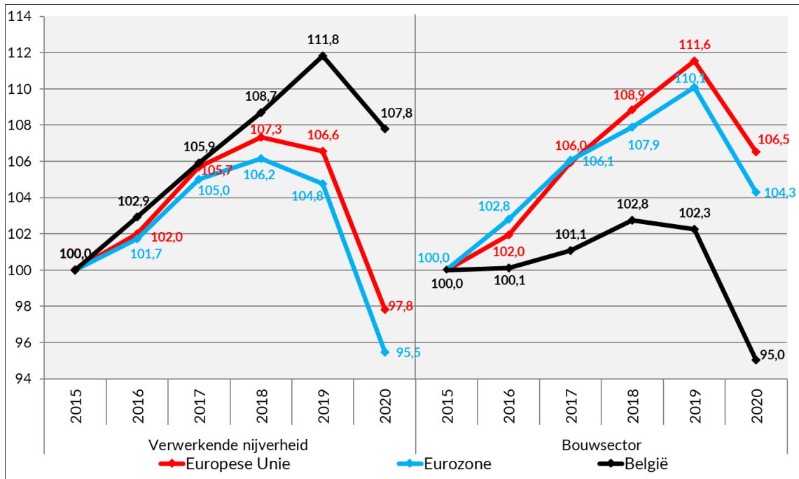
Grafiek 18. Productie-index in de verwerkende nijverheid en in de bouw Index 2015 = 100.
