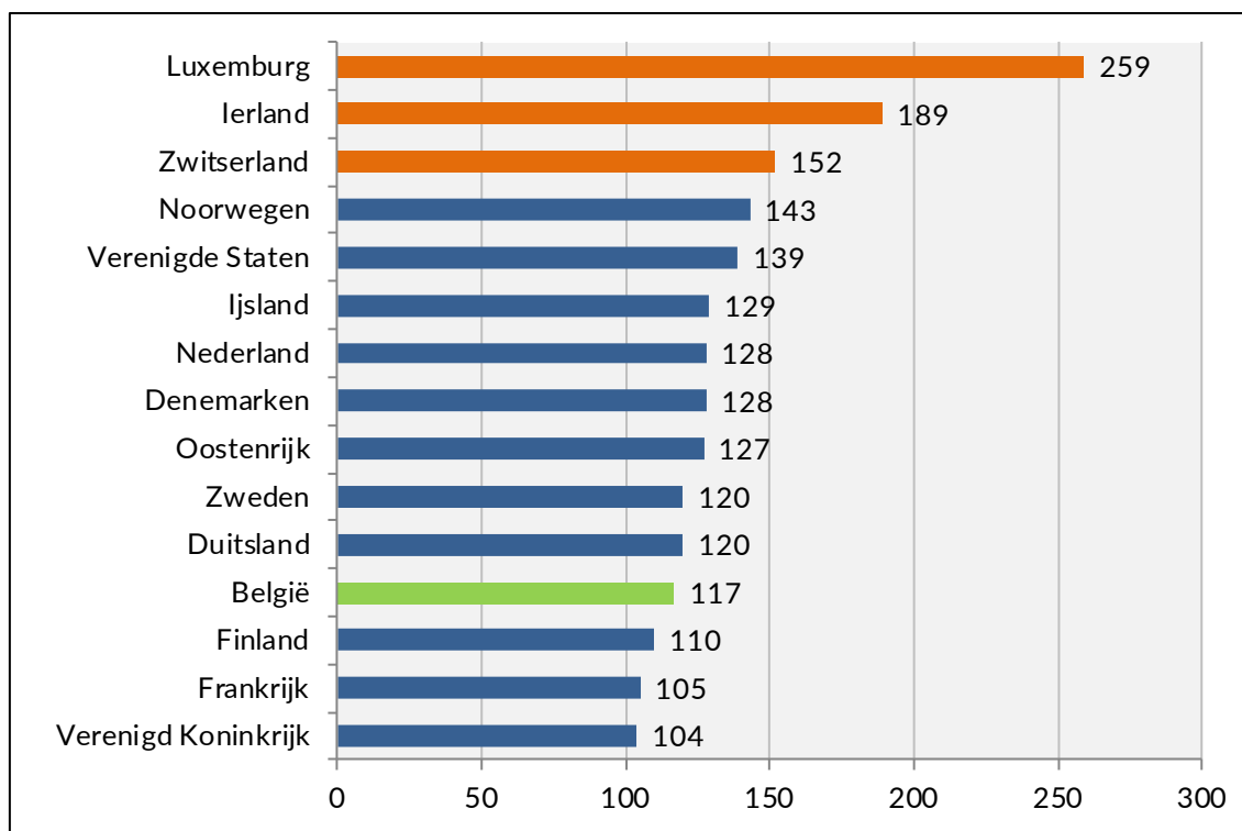
Grafiek 3. Bbp per inwoner, uitgedrukt in koopkrachtpariteit, in 2019 EU28 = 100.
