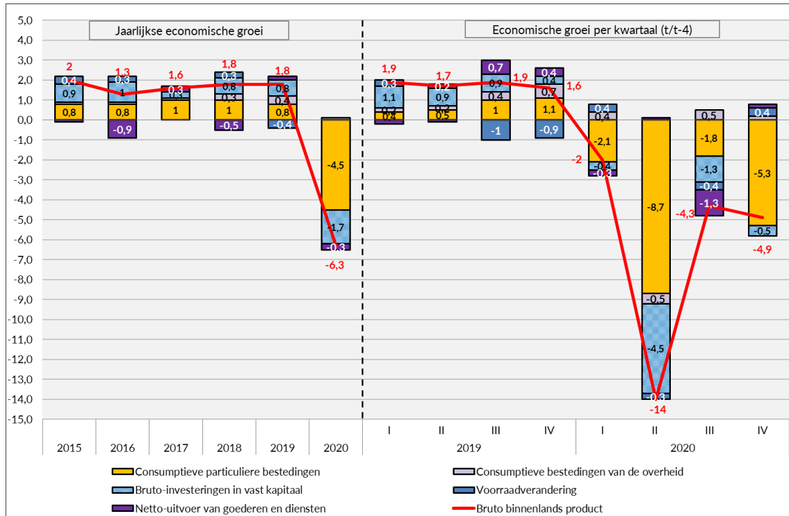
Grafiek 4. Evolutie van het bbp in % en bijdrage van de verschillende componenten vanuit uitgavenoptiek
