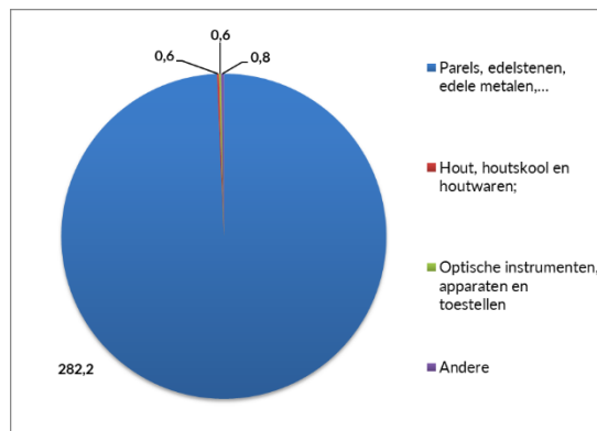
Grafiek 16. Invoer vanuit Angola in 2020 In miljoen euro.
