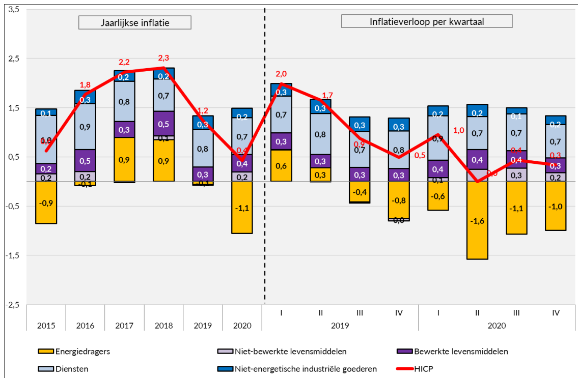
Grafiek 11. Evolutie van de geharmoniseerde consumptieprijsindex (HICP) en bijdrage aan de inflatie van de 5 grote aggregaten
