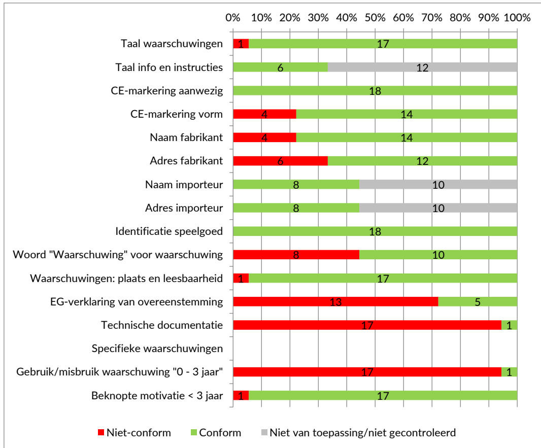
Grafiek 2. Resultaten van de controle van de administratieve vereisten (n=18)
